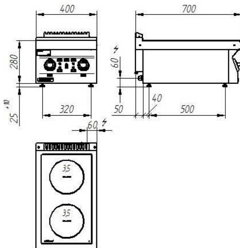
rys 2. Wymiary 700.KE-2i, 700.KE-2iF
