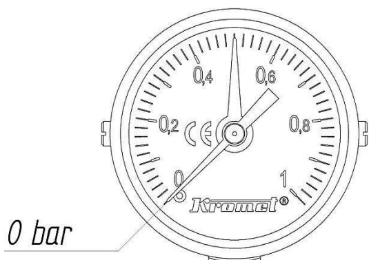
rys 8. Wskazanie manometru podczas gdy urządzenie jest wyłączone i ostudzone
