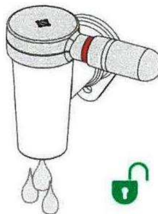
rys 21. Widok na zawór spustowy strawy w pozycji pełnego otwarcia
