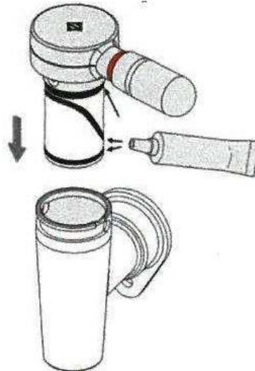
rys 27. Widok na zawór spustowy stawy w trakcie konserwacji tłoka.
