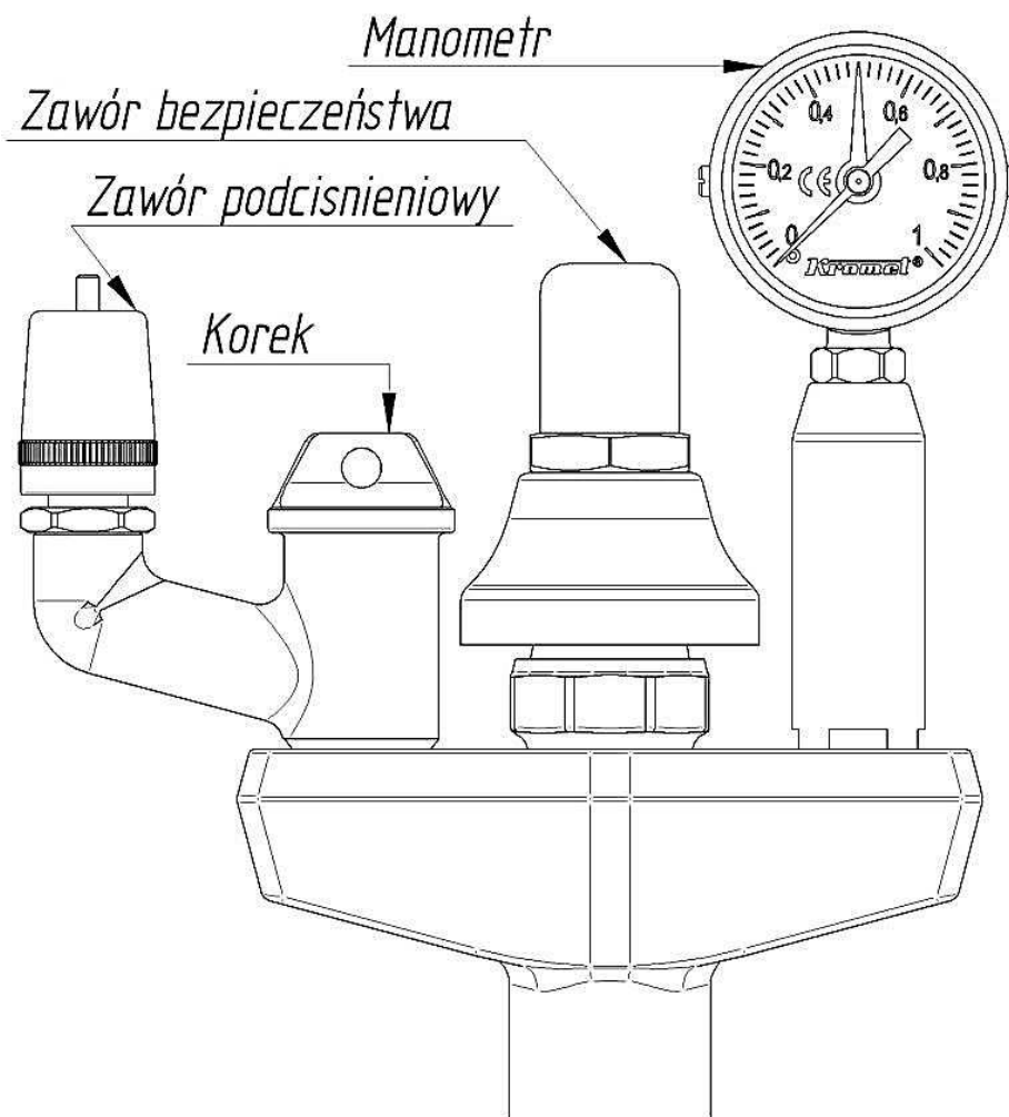
rys 7. Opis zespołu zabezpieczającego
