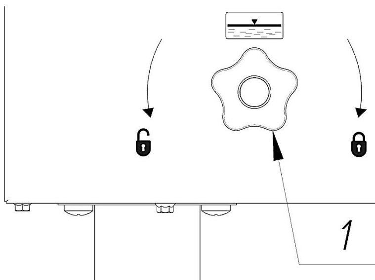
rys 12. Schemat usytuowania zaworu przelewowego
